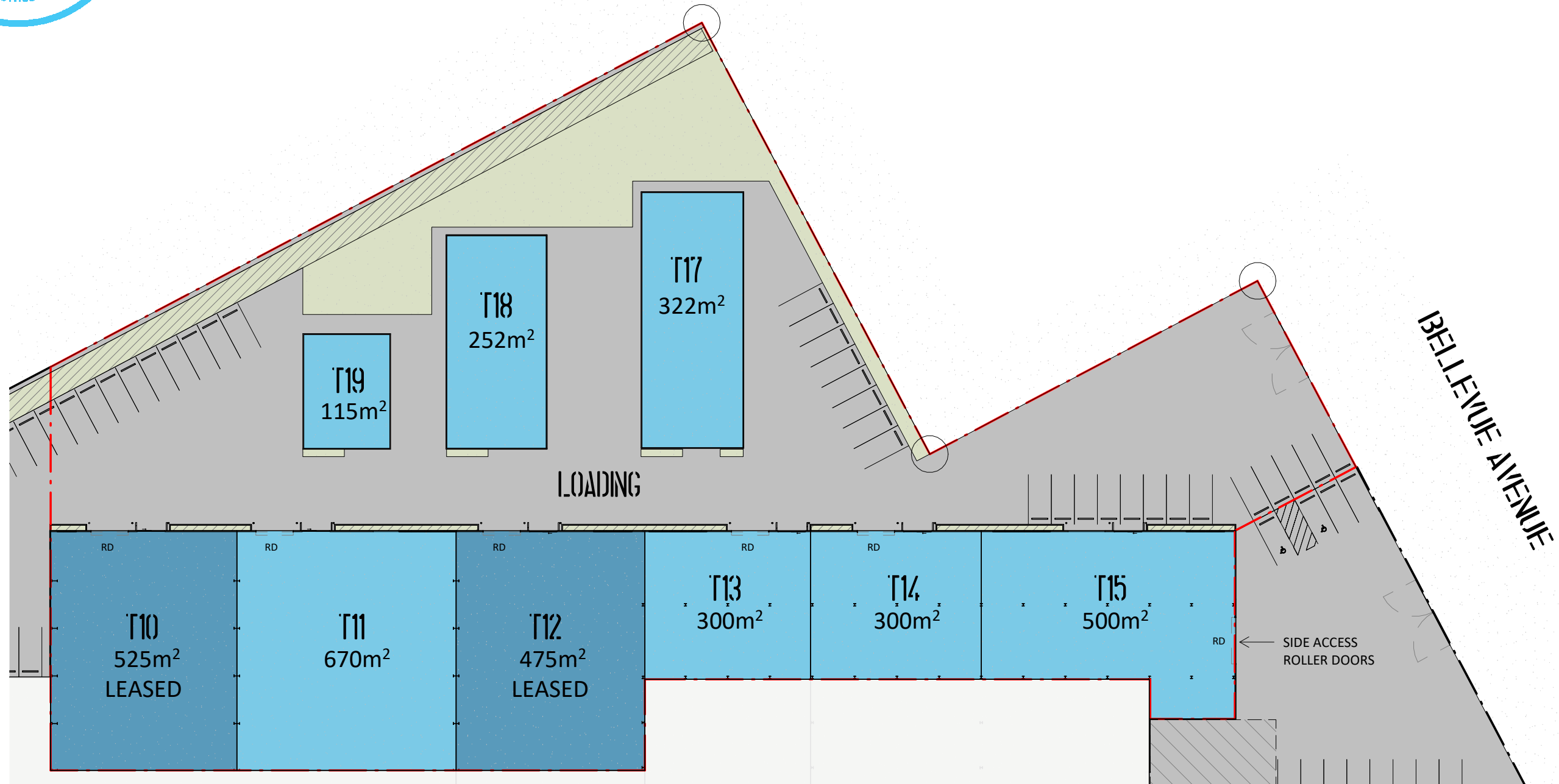
1 SITE PLAN - 88 BELLEVUE 1 : 500
