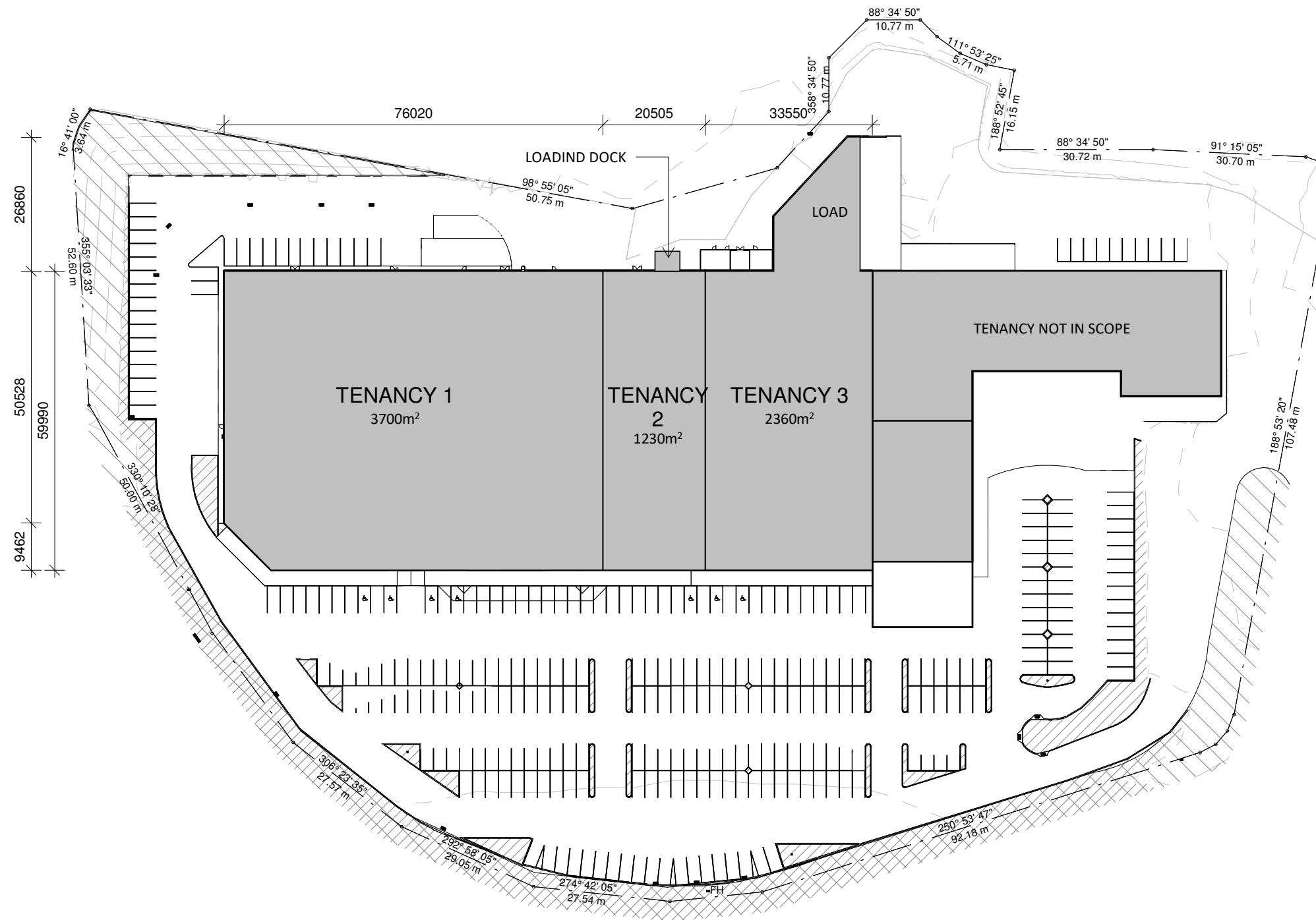
1 TENANCY PLAN 1 : 1000
